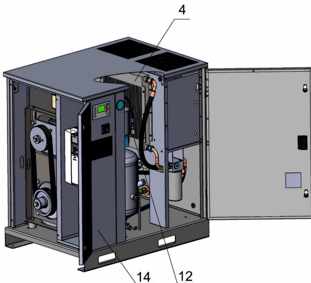
Рисунок 1.а – Общий вид компрессорной установки BK20T-8(10,16)
